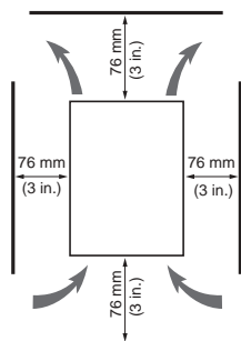
Figura 3: Espacio libre mínimo (575 V)
