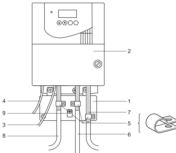
Figura 5: Diagrama de instalación
